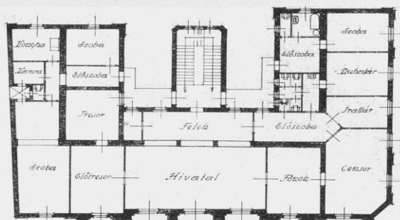
I. EMELETI ALAPRAJZ
